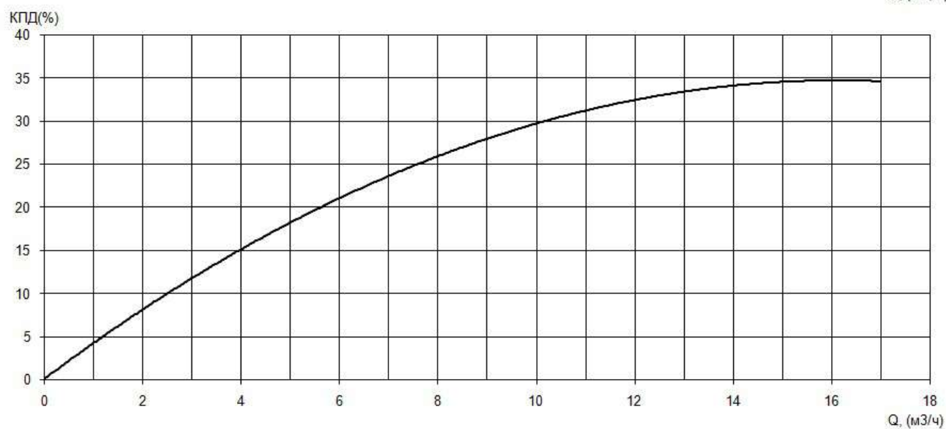
Рабочие характеристики насоса серии «Иртыш» ПФс 50/120.128-1,1/2Ех
