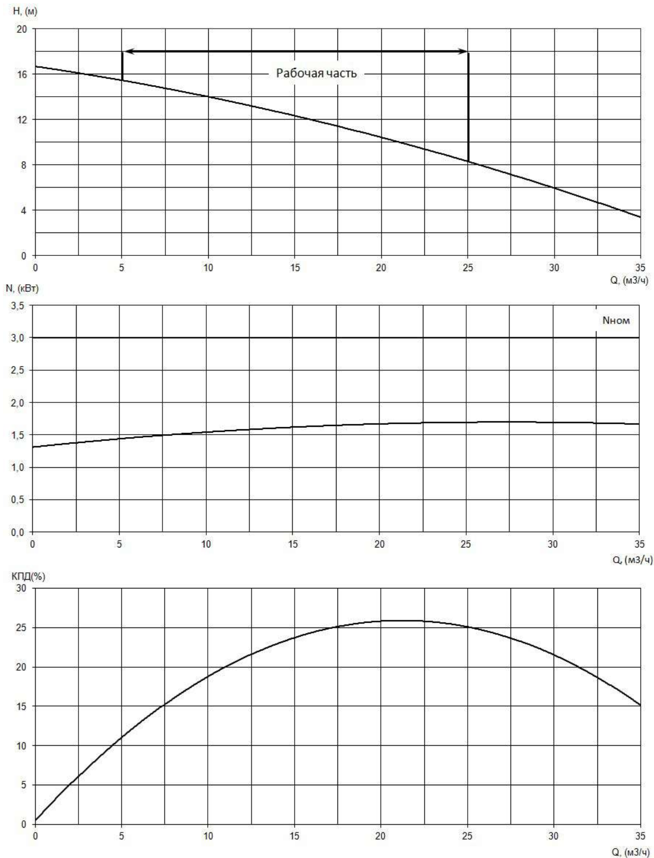
Рабочие характеристики насоса серии «Иртыш» ПФс 50/140.129-3/2Ех
