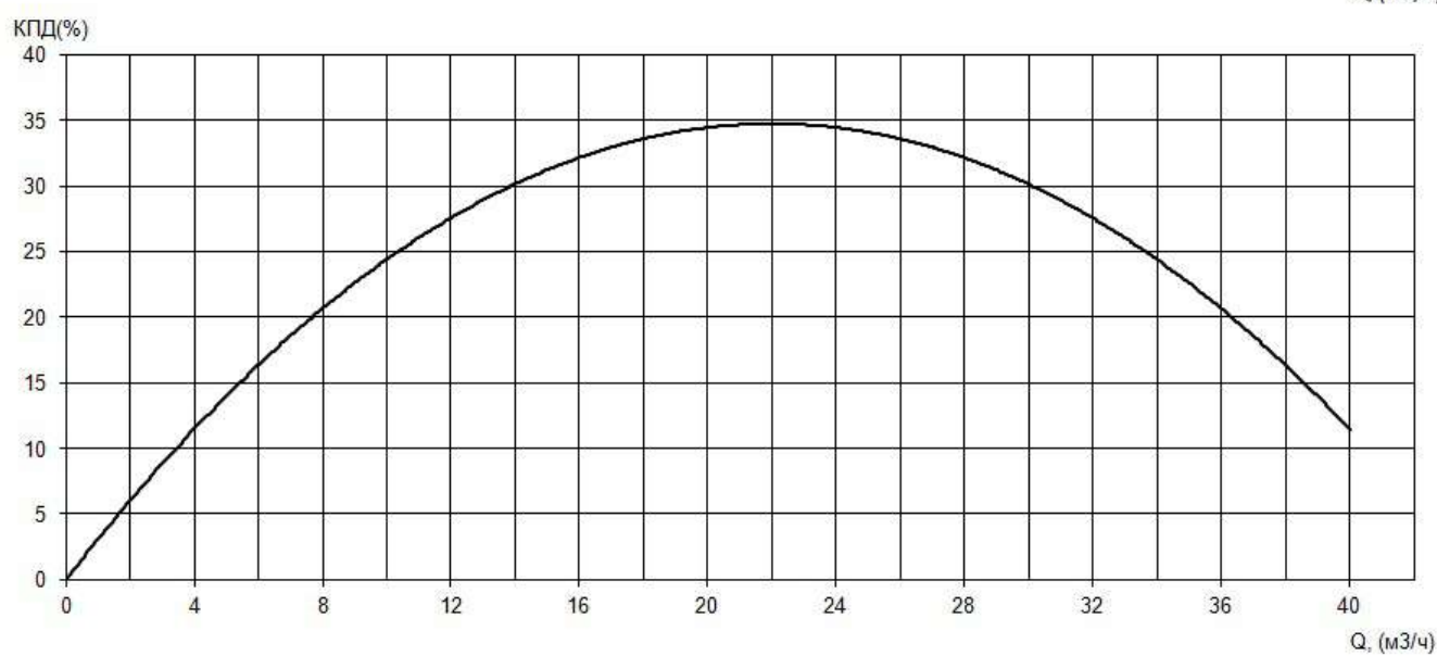
Рабочие характеристики насоса серии «Иртыш» ПФс 50/150.143-3/2Ex
