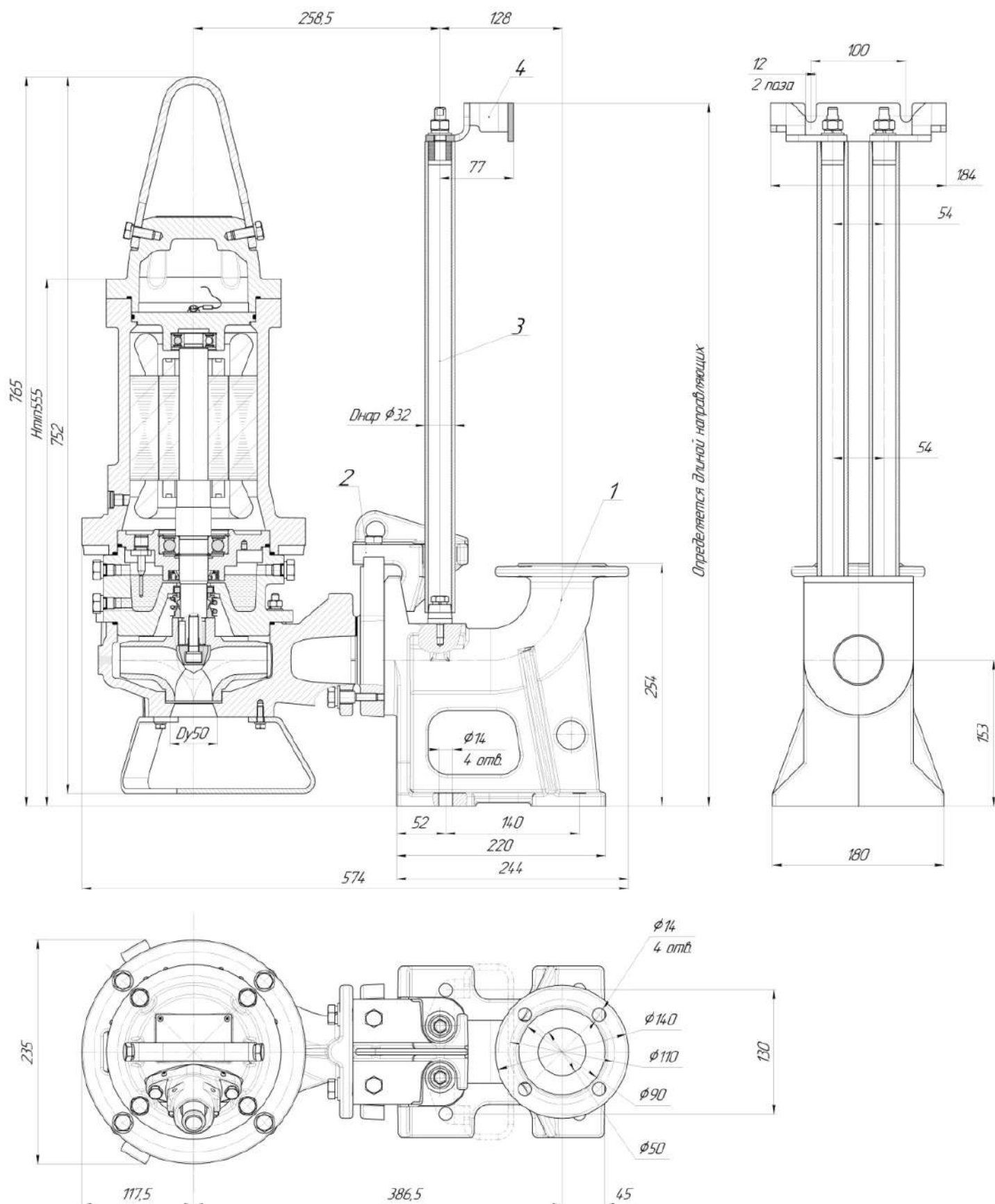
Общий вид и габаритные размеры электронасоса серии «Иртыш» ПФс 50/150.143-3/2Ex-106
